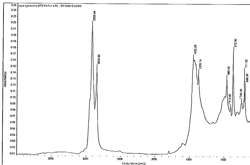
Rysunek 2 – Widmo w podczerwieni (analiza FTIR) – papa zgrzewalna EP5 Performa PL
